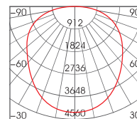
SAMSUNG 20W 80°
