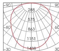
SAMSUNG 15W 80°
